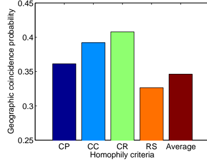
Fig. 3. Link Homophily
